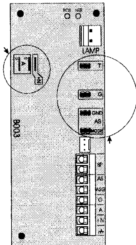
Obr. 2. Propojky na plošném spoji
